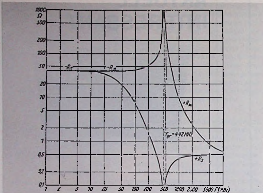
Bild 15. Frequenzabhängigkeit der Ersatzwiderstände R_s und R_n
