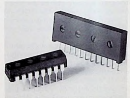
Trimmwiderstände und Widerstands-Netzwerke im DIL- oder SIL-Gehäuse (Preh)
