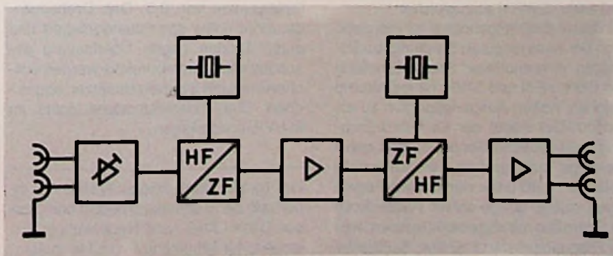
Bild 16. Blockschaltbild des UKW-Kanalumsetzers Lvu 8201 (Bilder: Hirschmann)
