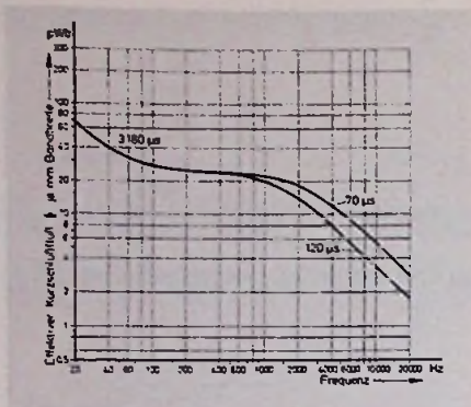
Bild 3. Frequenzgang des Bandflusses im Kurzschluß nach DIN 45 513 Teil 6 und Teil 7
