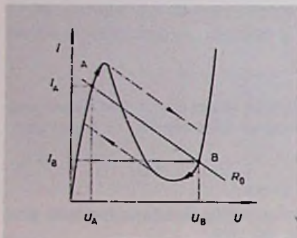
Bild 20. Arbeitskennlinie einer Tunnel diode für den Schaltbetrieb (SEL)
