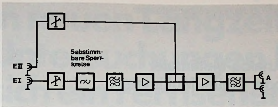
Bild 15. Blockschaltbild des Trennverstärkers LvB 3210
