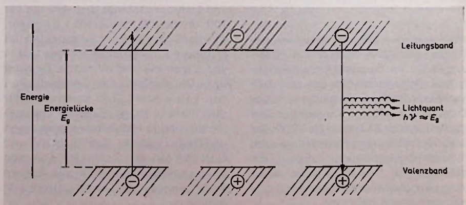
Bild 4. Energiebänder-Diagramm für eine LED
