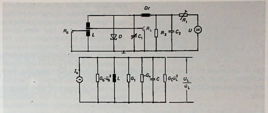
Bild 18. Selektiver HF-Verstärker mit einer Tunnelodiode und gleichstrommäßiger Parallelspeisung oben: Schaltung unten: Ersatzschaltbild
