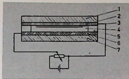
Bild 18. Grundsätzlicher Aufbau eines elektrochromen Displays. 1 transparentes Substrat, 2 transparente Elektrodenschicht, 3 elektrochemische Schicht ( WO_3 ), 4 Elektrolyt, 5 Verschuß, 6 Grundelektrode, 7 Grundsubstrat
