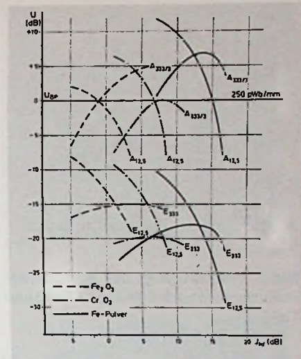
Bild 2. Elektroakustische Kennlinien von Cassettentonbändern
