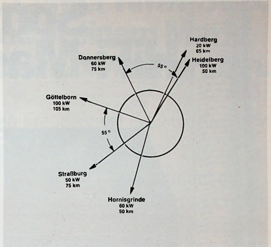
Bild 12. Anlagen-Beispiel „Karlsruhe“ mit Rundempfangsantenne
