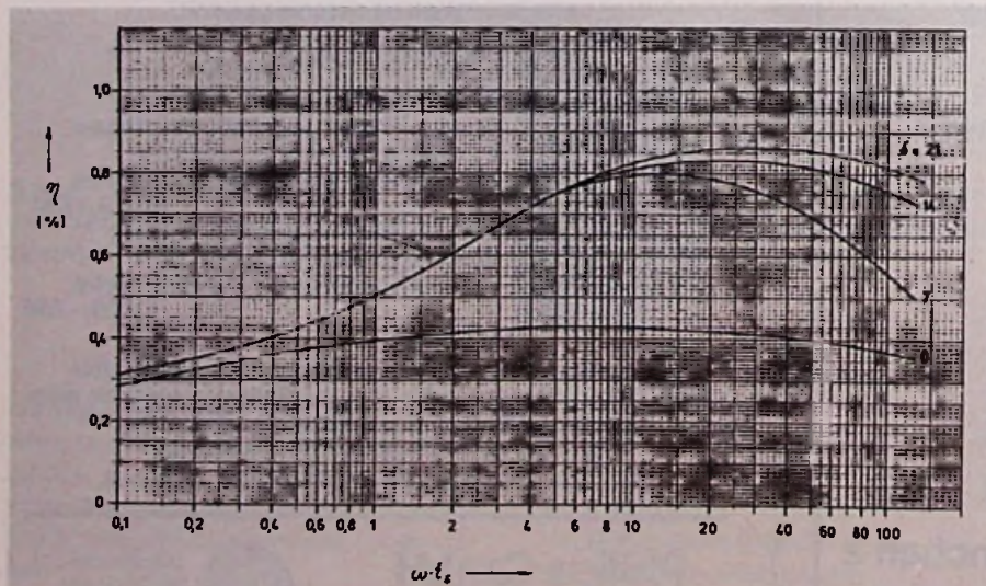
Bild 10. Maximaler Wirkungsgrad des Frequenzverdopplers mit realer Speicherschaltodiode bei Aussteuerung von U_B bis zum Optimum in Flußrichtung; Q = 100 ; n = 0,1 (nach Unger/Harth)
