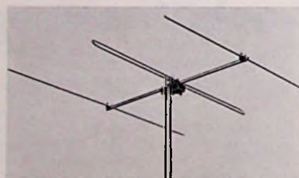
Bild 5. UKW-3-Elementantenne
