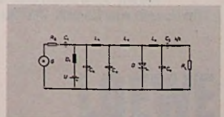
Bild 5. Prinzipschaltbild eines Frequenzvervielfachers mit einer Speicher-Schaltdiode
