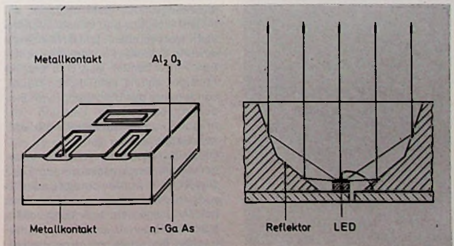
Bild 6. Querschnitt durch ein monolithisches (links) und ein diskretes (rechts) LED-Display
