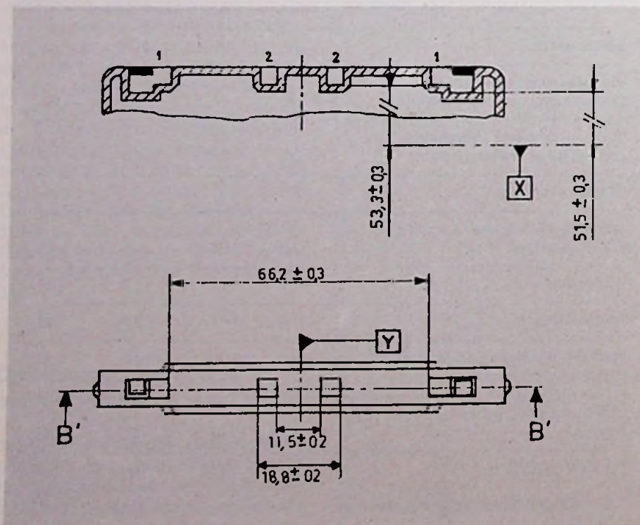
Bild 4. Vorschlag zum automatischen Umschalten bei Eisenpulver-Cassetten
