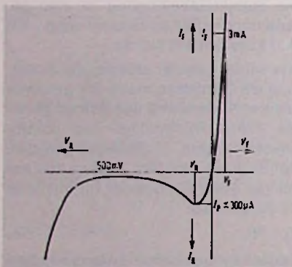
Bild 21. Strom-Spannungskennlinie der Backward-Diode TU 300 (Siemens)
