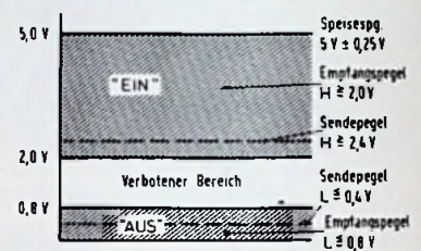
Bild 1.2. Zuordnung von Toleranzfeldern für die Zustände „ein“ und „aus“ bei TTL-Digitalschaltungen
