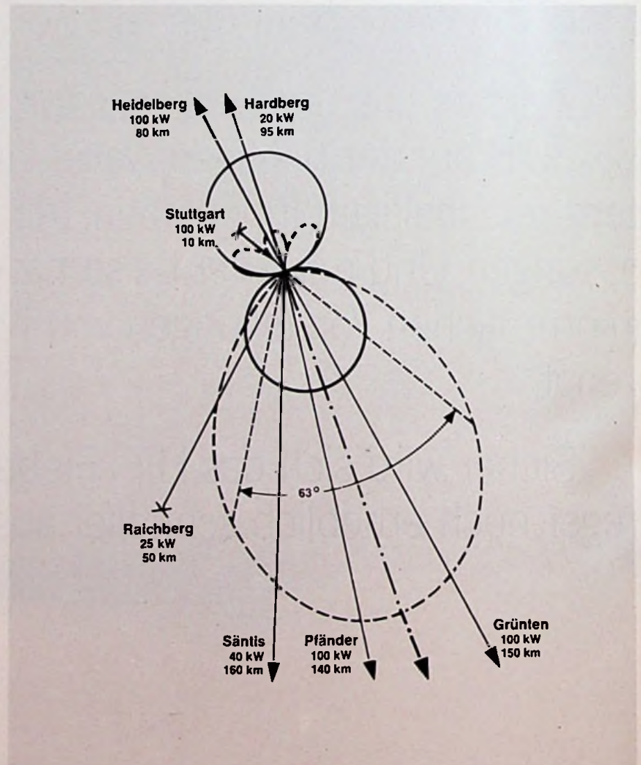
Bild 14. Anlagen-Beispiel „Nellingen“ mit einfachem Dipol und Richtantenne
