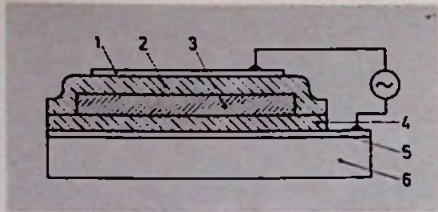
Bild 19. Grundsätzlicher Aufbau eines (AC)-Elektrolumineszenz-Displays. 1 Al, 2 Y 2 O 3 , 3 ZnS:Mn, 4 Y 2 O 3 , 5 SnO 2 , 6 Glas
