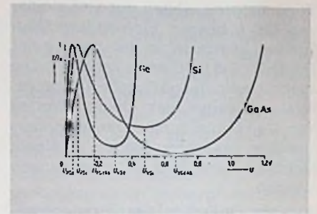
Bild 13. Strom-Spannungskennlinien von Tunnelndioden aus verschiedenen Materialien (Siemens)
