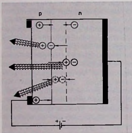
Bild 3. LED-Chip mit Lichtemission am pn-Übergang
