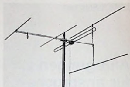
Bild 7. UKW-5-Elementantenne
