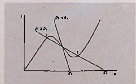
Bild 17. Statische Stabilitätsbedingungen
