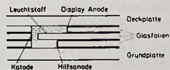
Bild 14. Flacher Plasma-Bildschirm mit positiver Säule. Querschnitt durch eine Zelle (oben) sowie schematische Anordnung und Betrieb der Zellen (unten). 1 Display-Anode, 2 Hilfsanode, 3 Katode, 4 Widerstand, 5 Display-Gasentladungsraum, 6 Hilfs-Gasentladungsraum
