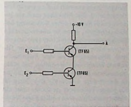
Bild 3.1. Beispiel einer negativen Logik (NAND) mit PNP-Transistoren
