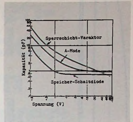
Bild 4. Verlauf der Kapazität verschiedener Diodentypen in Abhängigkeit von der Spannung (Alpha)
