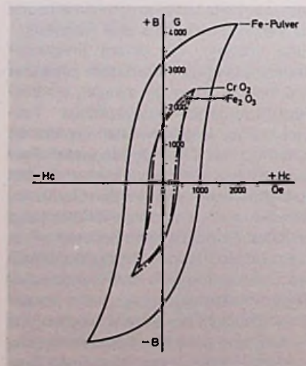
Bild 1. Hystereseschleifen von Cassettentonbändern. 1 \text{ G} = 10^{-4} \text{ T} , 10 \text{ Oe} \approx 0,8 \text{ A/cm}
