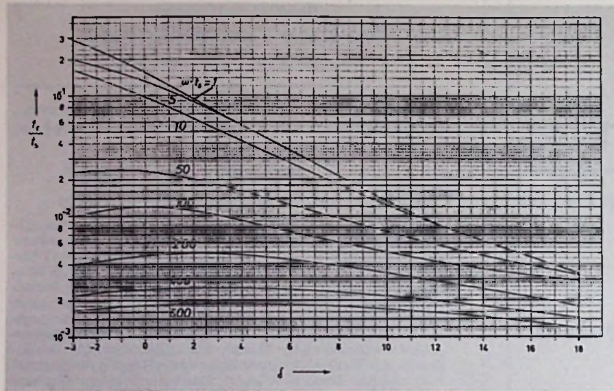
Bild 9. Driftkonstante \delta in Abhängigkeit vom Verhältnis t_r/t_s für verschiedene Werte von \omega \cdot t_s (nach Unger/Harth)
