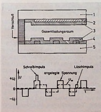
Bild 12. Grundsätzlicher Aufbau einer AC-Plasmaanzeige im Querschnitt (oben) und das Ansteuerschema (unten). 1 Glasplatte, 2 x-Leiter, 3 Dielektrikum, 4 y-Leiter, 5 Glasplatte, U_w Wandspannung, U_i Zündspannung
