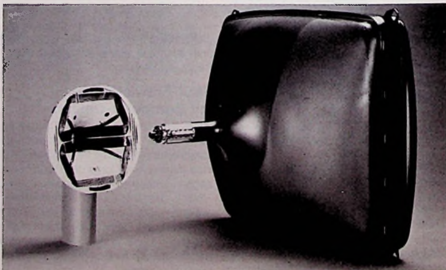
Bild 1. Das Farbbild-System 30 AX von Valvo besteht aus der Ablenkeinheit und der Bildröhre, an deren Konus die drei Paßauflagepunkte zu erkennen sind
