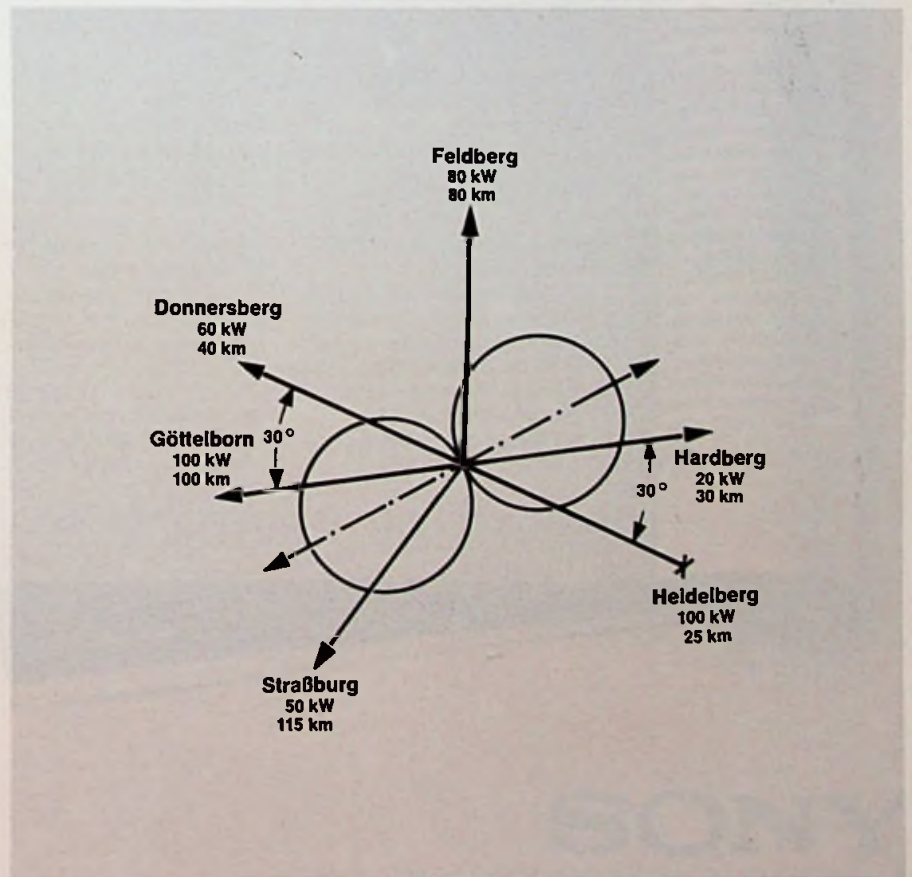
Bild 13. Anlagen-Beispiel „Ludwigshafen“ mit einfachem Dipol
