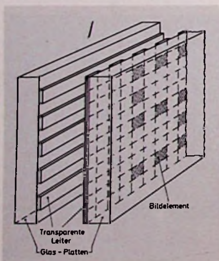
Bild 8. Grundsätzlicher Aufbau eines Plasmadisplays
