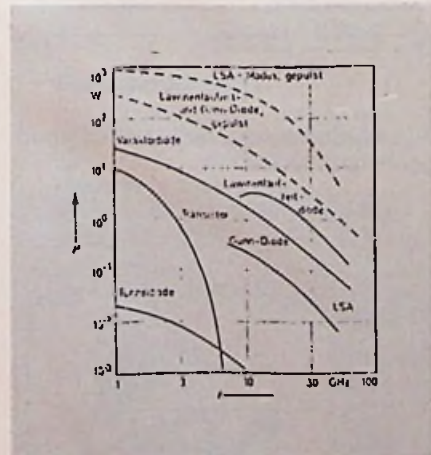
Bild 14. Frequenz-Leistungskurven von Mikrowellengeneratoren
