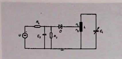
Bild 19. Selektiver HF-Verstärker bzw. Oszillator (ohne Koppelwicklungen) und gleichstrommäßiger Serienschaltung
