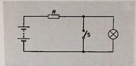
Bild 2.3. Mit der NICHT-Verknüpfung leuchtet die Glühlampe bei offenem Schalterkontakt auf
