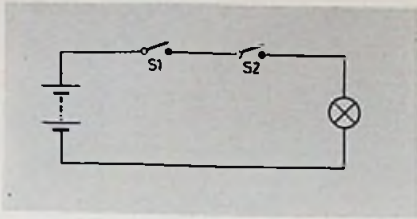
Bild 2.1. Erklärung einer UND-Verknüpfung anhand einer Kontaktschaltung mit angeschlossener Glühlampe
