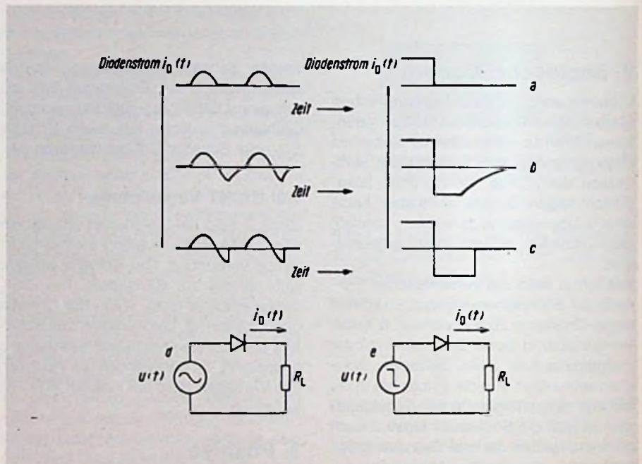
Bild 2. Verlauf der Diodenströme verschiedener Dioden bei Ansteuerung mit einer Sinus- und einer Rechteckspannung (Siemens). a ideale Diode, b herkömmliche Schaltdiode, c Speicher-Schaltdiode, d, e Meßschaltungen
