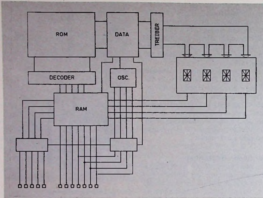
Bild 7. Schaltung eines intelligenten Displays
