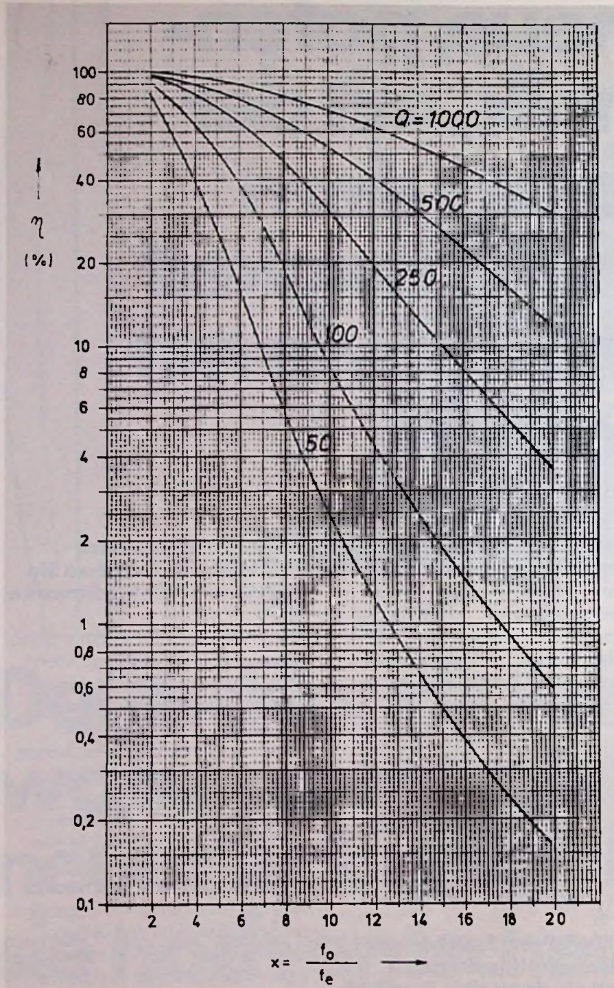
Bild 6. Wirkungsgrad \eta einer idealen Speicher-Schaltodiode in Abhängigkeit vom Vervielfachungsfaktor x bei unterschiedlichen Diodengüten Q (nach Unger/Harth)
