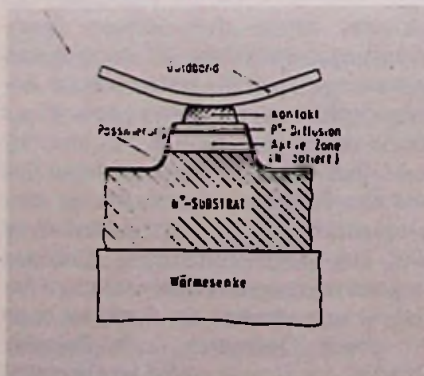
Bild 1. Schnittbild durch den Aufbau einer Speicher-Schaltdiode (Siemens)
