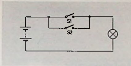
Bild 2.2. Erklärung einer ODER-Verknüpfung anhand einer Kontaktschaltung mit angeschlossener Glühlampe
