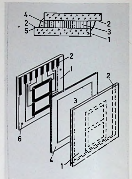
Bild 16. Querschnitt durch eine Flüssigkristallzelle (oben) und ihr Aufbau (unten). 1 Glasplatte, 2 Elektroden-schicht, 3 Flüssigkristall, 4 Abstandsrahmen, 5 Verschluss, 6 Füllöffnung
