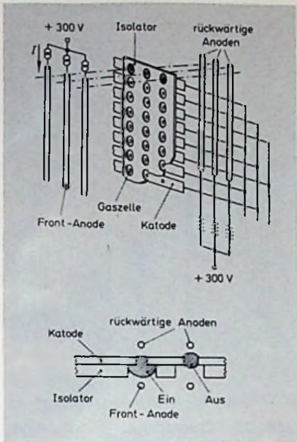
Bild 11. Grundsätzlicher Aufbau einer DC-Plasmaanzeige mit Schiebebetrieb
