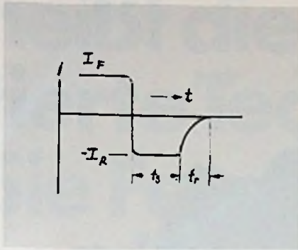
Bild 3. Zeitlicher Verlauf des Diodenstromes einer Speicher-Schaltdiode beim Umschalten vom Durchlaßgebiet in das Sperrgebiet
