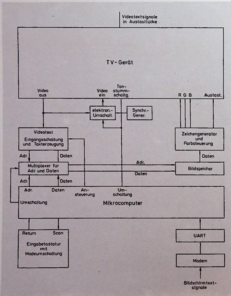
Bild 3. Blockschaltbild Videotext-Bildschirmtext-Empfängergerät
