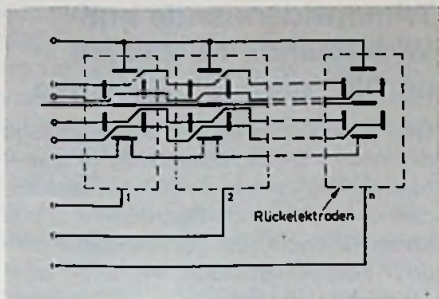
Bild 17. Verbindungsschema von 7-Segment-Anzeigen für 7-Schritt-Multiplexbetrieb
