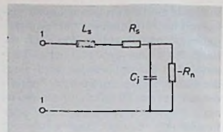
Bild 16. Ersatzschaltbild der Tunnel diode
