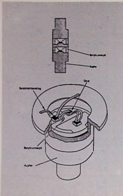
Bild 11. Serienschaltung mehrerer Speicher-Schaltdioden durch Aufeinanderstapeln (a) oder durch Anbringen in einer Ebene (b) zum Erzielen einer höheren Durchbruchsspannung (Siemens)
