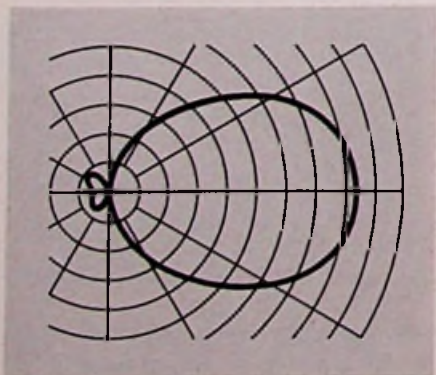
Bild 6. Richt-Diagramm der UKW-3-Elementantenne
