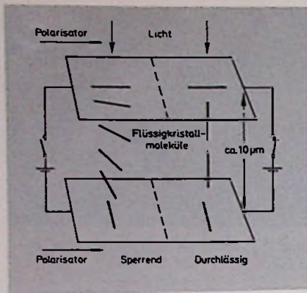
Bild 15. Grundsätzlicher Aufbau einer Schadt-Helfrichzelle
