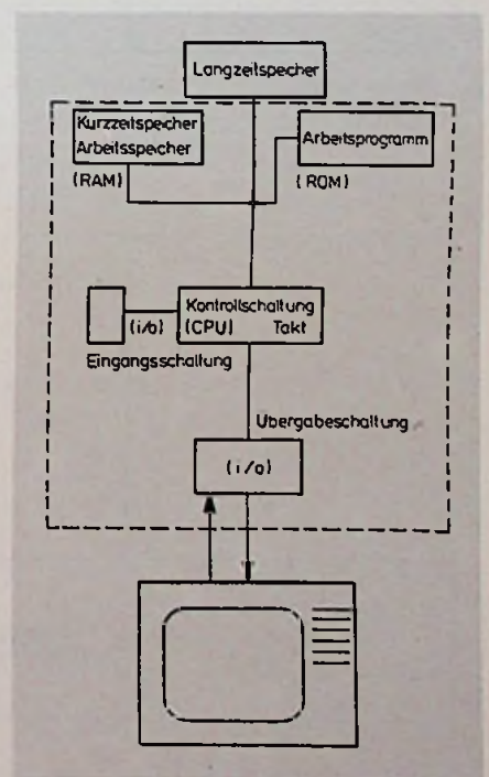
Bild 1. Schematischer Aufbau eines Bedienteils
