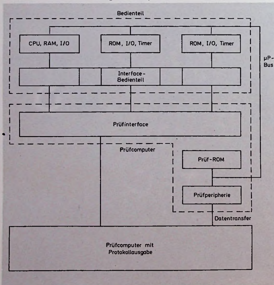
Bild 2. Prüfaufbau für die Prüfung von Mikroprozessor-Bedienteilen
