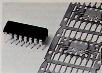
DIL-Gehäuse mit Kupferrahmen zum Abführen hoher Verlustleistungen (SGS-Ates)
